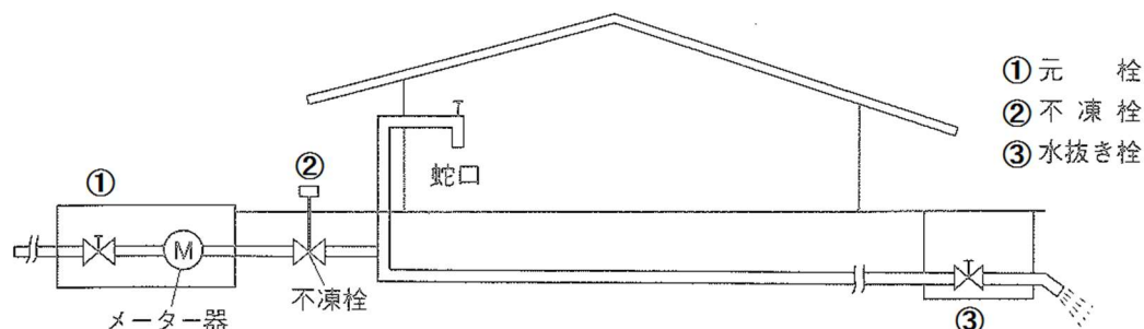
水抜き設備例
